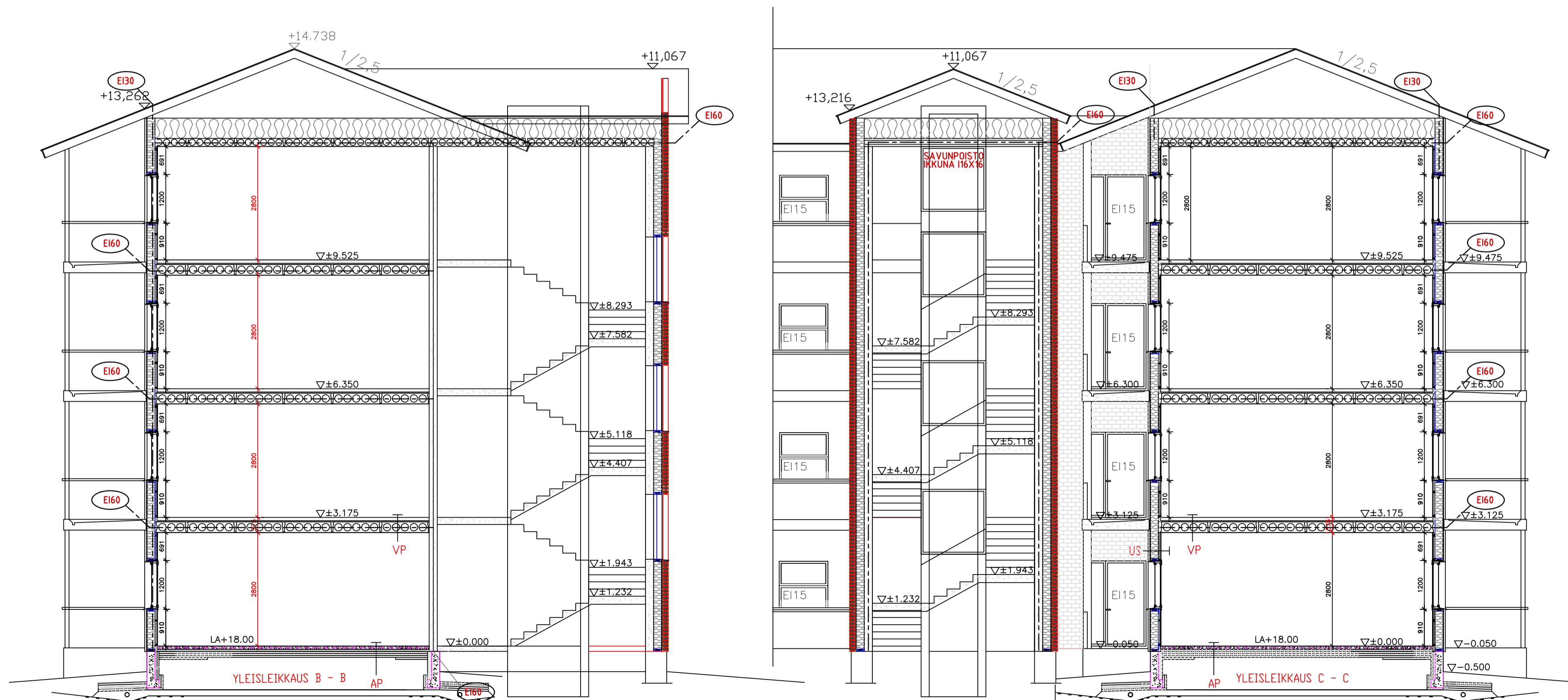
PERUSTUKSET RAKENNESUUNNITELMIEN MUKAAN
